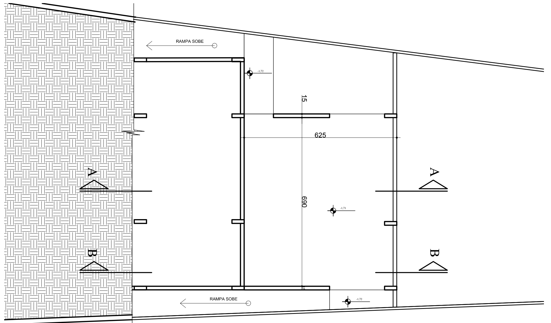
PLANTA BAIXA - NÍVEL -1,71 Esc: 1/75 ÁREA = 45,01m 2
