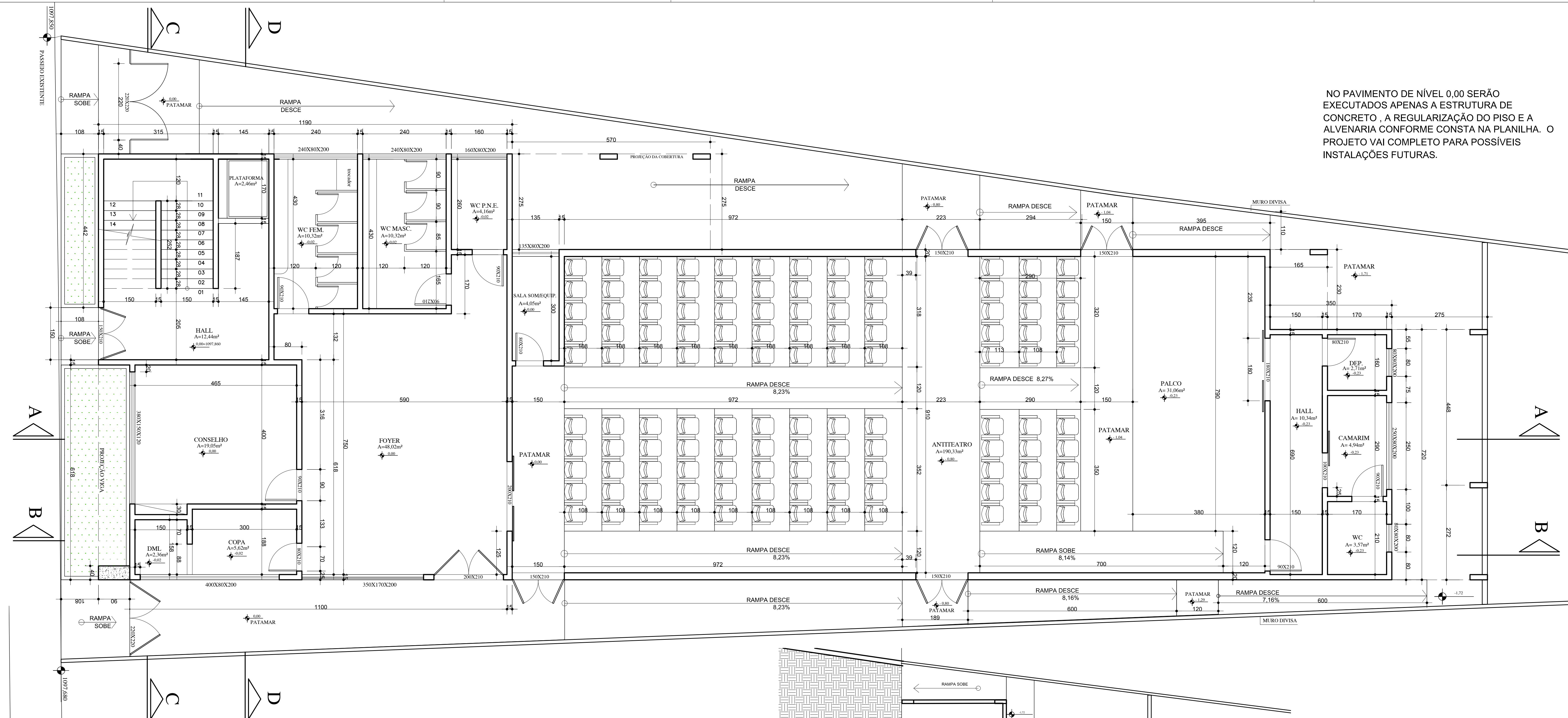
PLANTA BAIXA - NÍVEL 0,00 Esc: 1/50 ÁREA = 411,78m 2
