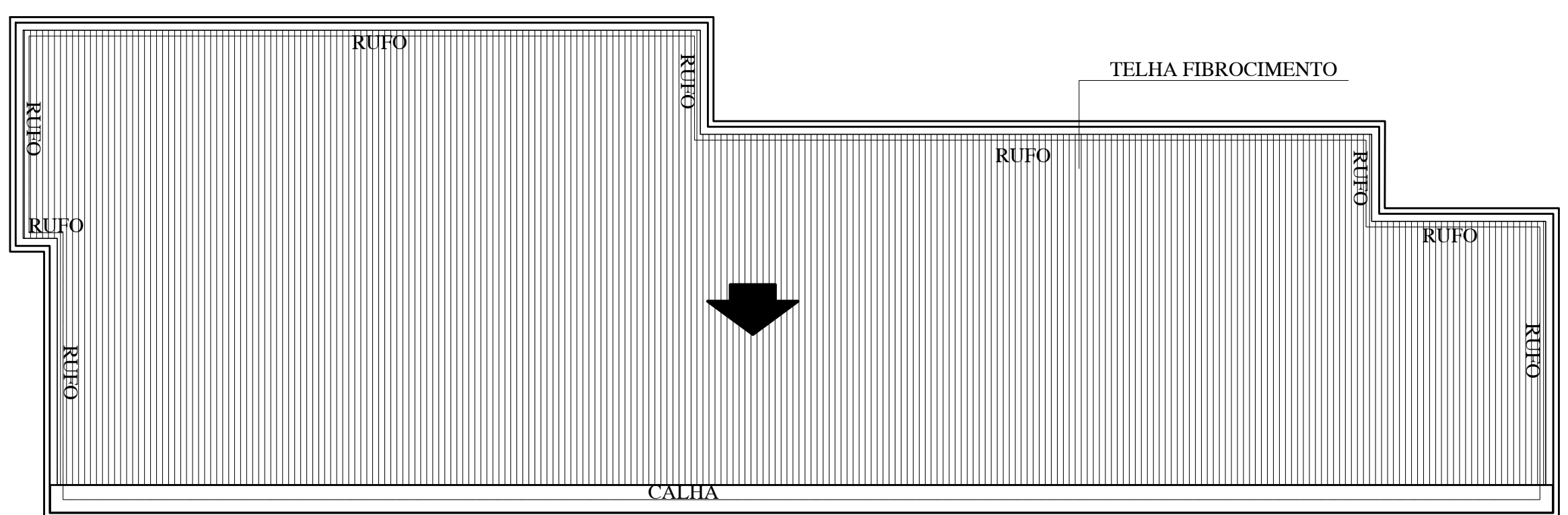
PLANTA COBERTURA Esc: 1/125
